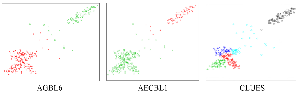
Figura 5.7: Comparação entre os agrupamentos obtidos por AGBL6, AECBL1 e CLUES para a instância 300p2c1 [11].
