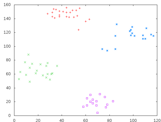
Figura 5.3: Solução gerada para ruspini com o algoritmo AGBL6.
