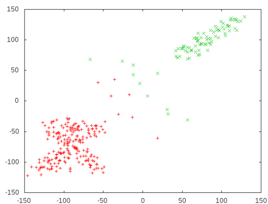
Figura 5.5: Solução gerada para 300p2c1 com o algoritmo AGBL6.
