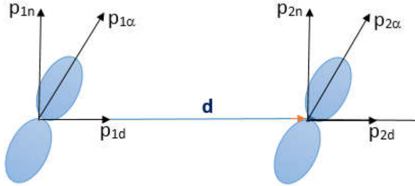
Figura 1.9: Ligações entre Orbitais P
