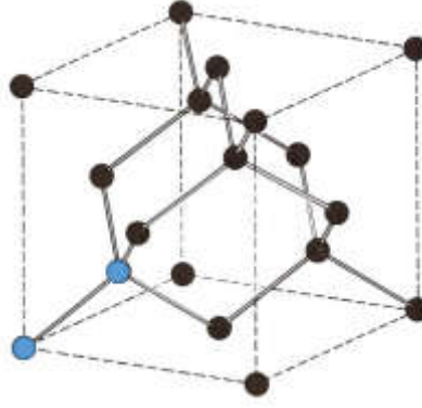
Figura 1.5: Célula Primitiva do Silício
