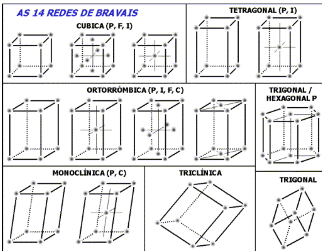
Figura 1.2: As redes de Bravais - Imagem retirada de [Aguar Junior, 2006]
