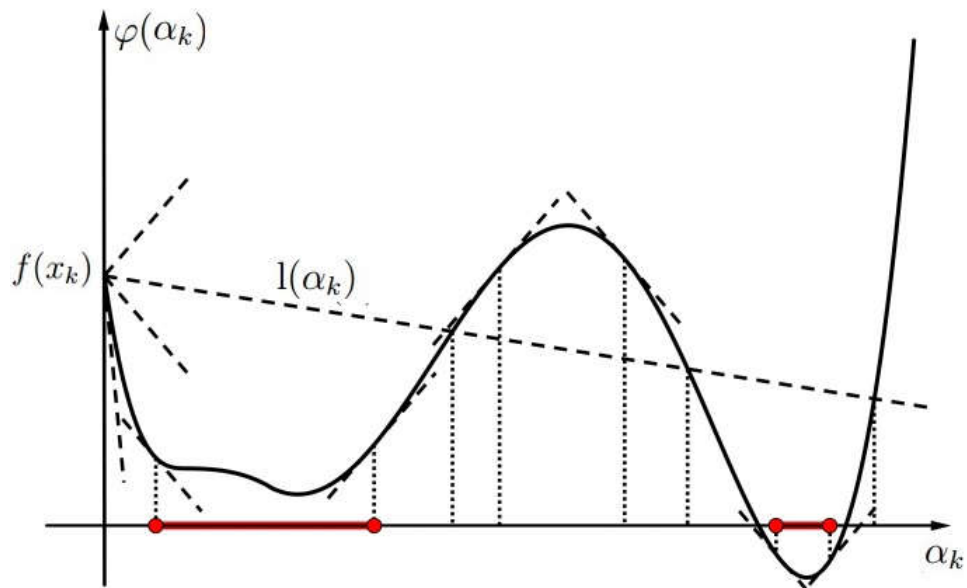
Figura 2.4: Valores de \alpha_k que satisfazem a Condição de Curvatura
