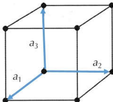
Figura 1.1: Vetores Primitivos em um Cristal
