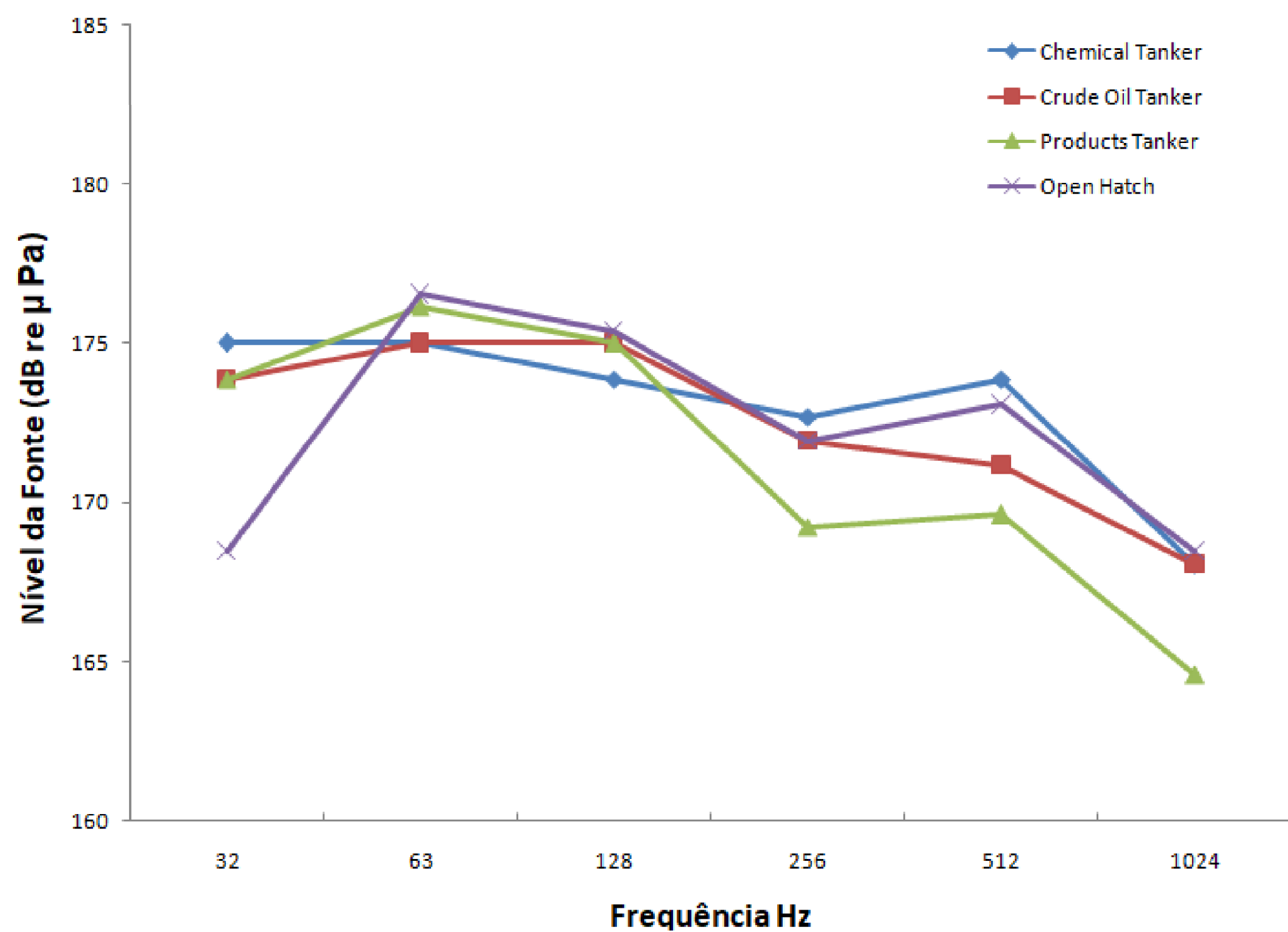
Figura 5.10 – Níveis acústicos e frequências para os navios Chemical Tanker , Crude Oil Tanker , Products Tanker e Open Hatch - Adaptado de McKenna et al. (McKenna et al. , 2012).
