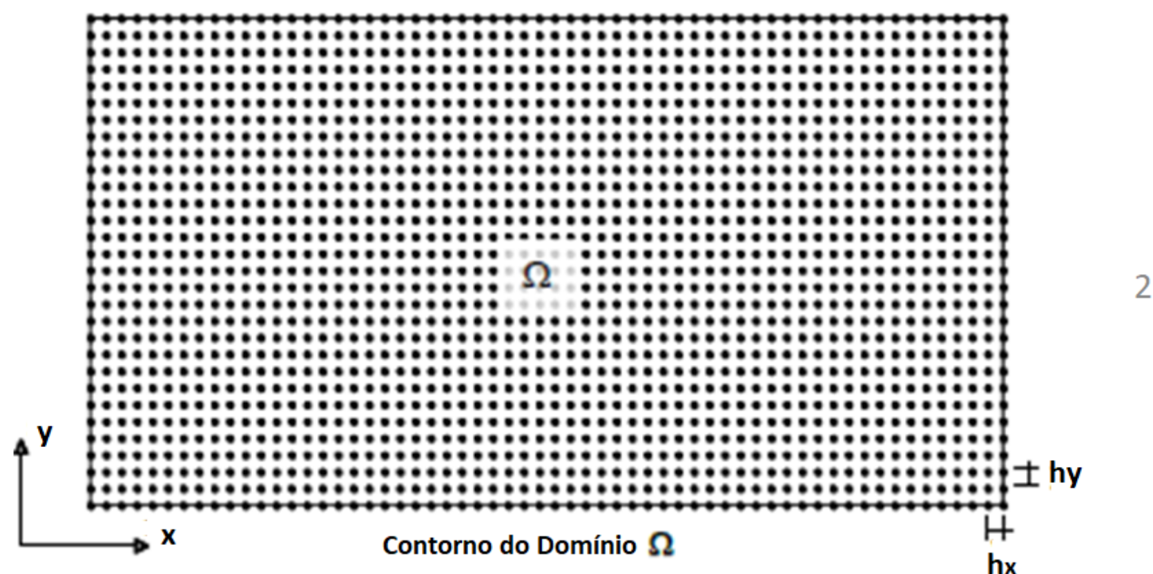
Figura 3.1 – Ilustração de uma malha bidimensional sobre domínio \Omega .
