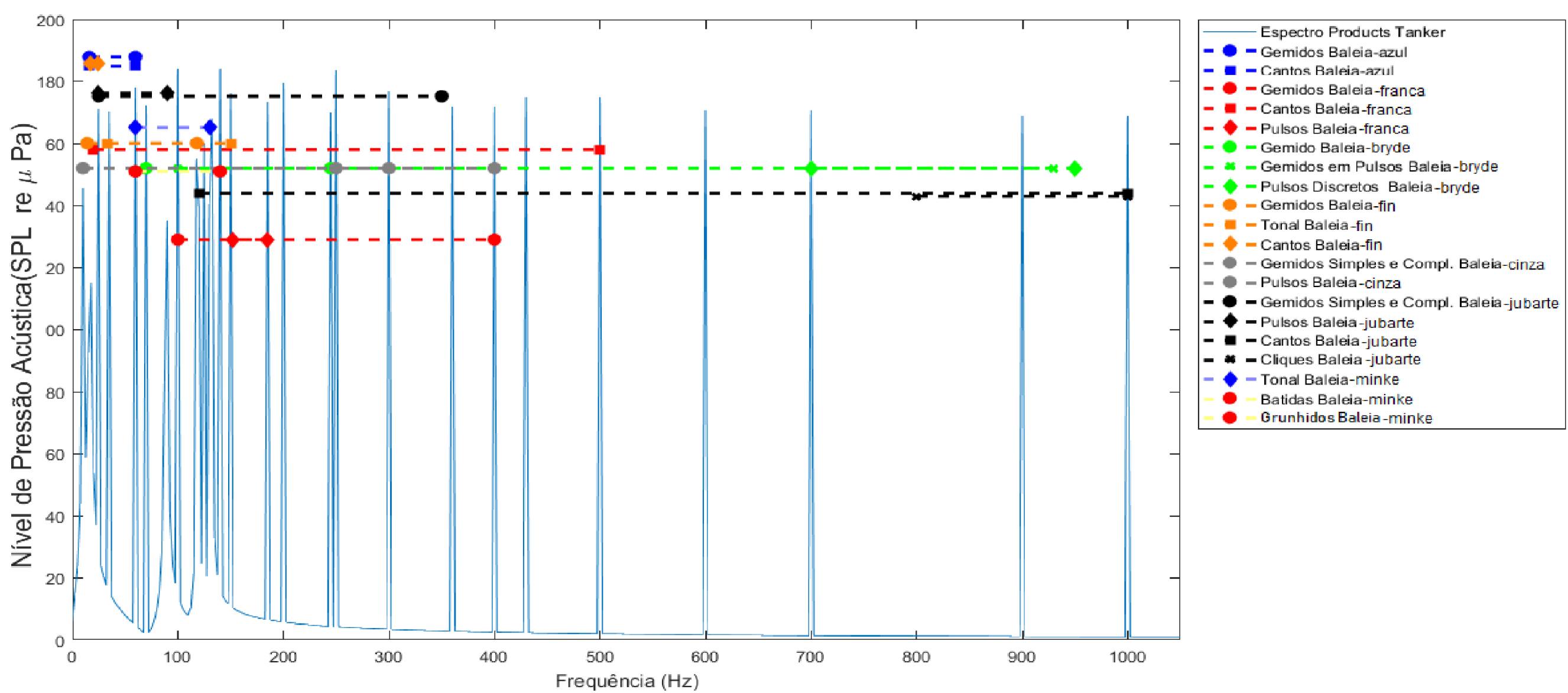
Figura 6.9 – Espectro dos sinais das fontes dos navios e faixas de frequência de vocalização dos mysticetos considerados neste trabalho.
