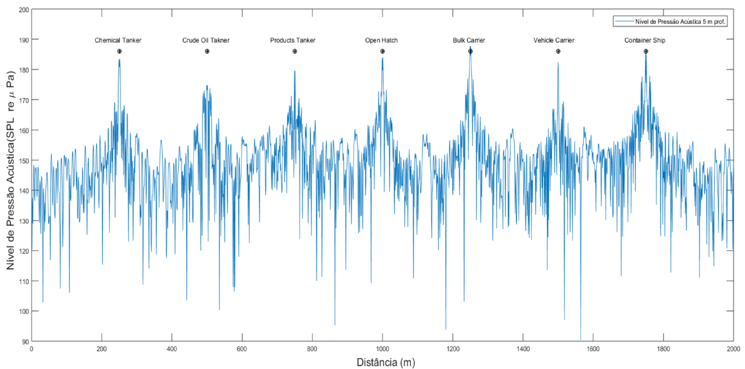
Figura 6.8 – Seção transversal da variação dos níveis de ruídos gerados por todas as classes de navio com as frequências dos mysticetos.
