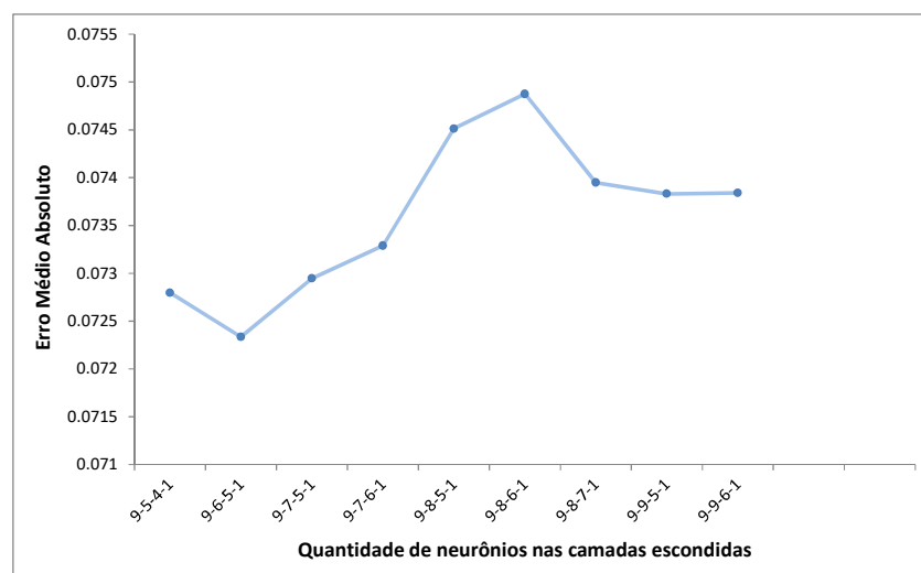
Figura 31 – Primeiro experimento do comportamento do erro MAE para diferentes quantidades de neurônios nas camadas escondidas
