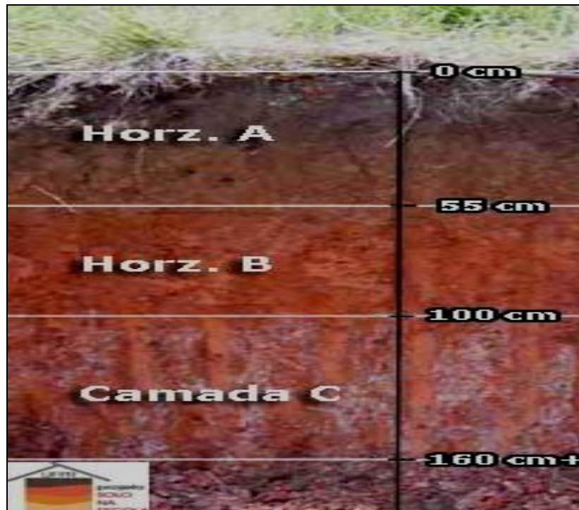
Horizontes do solo: Perfil de solo localizado em Pinhais (PR)
